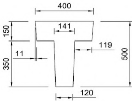
SECCIÓN VHPREF-50
