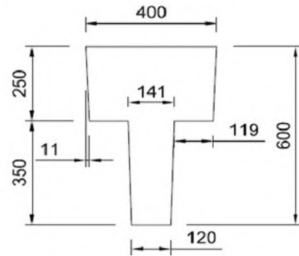
SECCIÓN VHPREF-60
